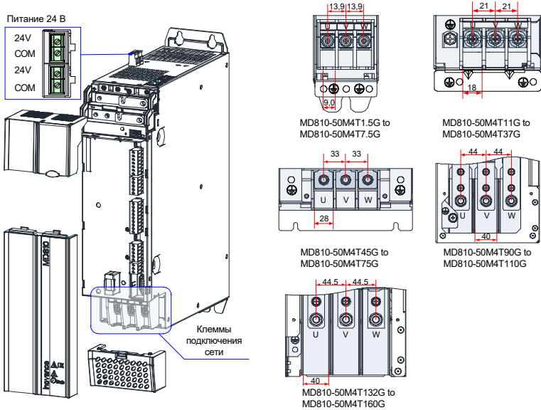
Рис. 3-1 Расположение клемм питания и размер модуля инвертора (одноосевой)
