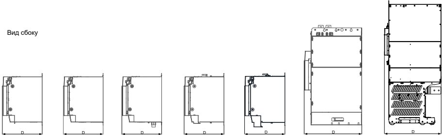
Рис. 1-3 Габаритные размеры модуля инвертора (одноосевой)
