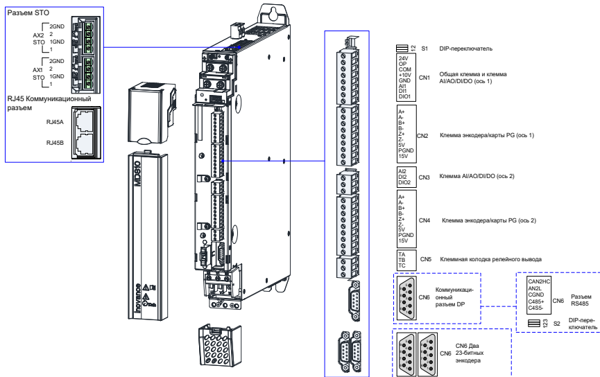
Рис. 3-5 Расположение клемм цепи управления модуля инвертора (двухосевой)
