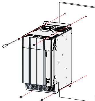
Рис. 2-3 Установка на монтажную панель MD810-50M4T45G–MD810-50M4T75G
